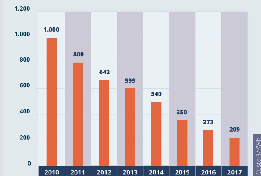
Evolução do custo de baterias lítio-íon 2010-2017 (US$/KWh)
