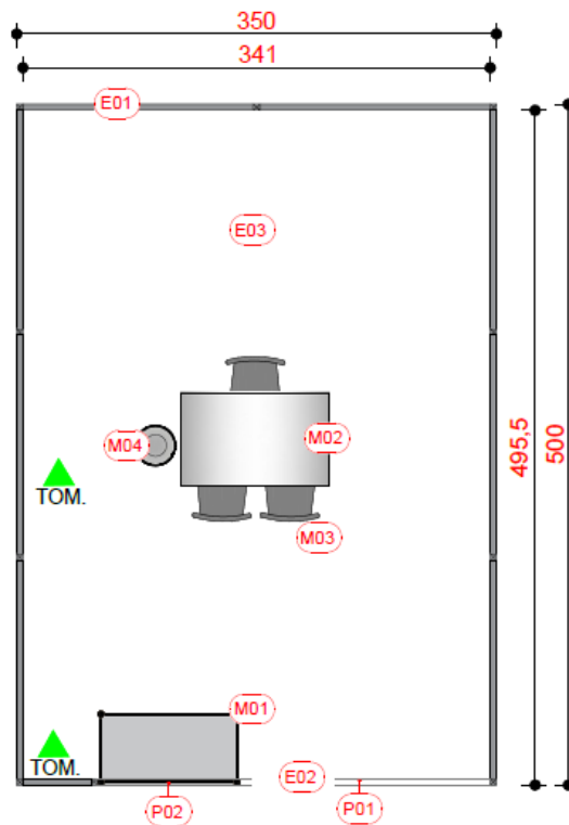
PLANTA ESTANDE - 17,5m 2
